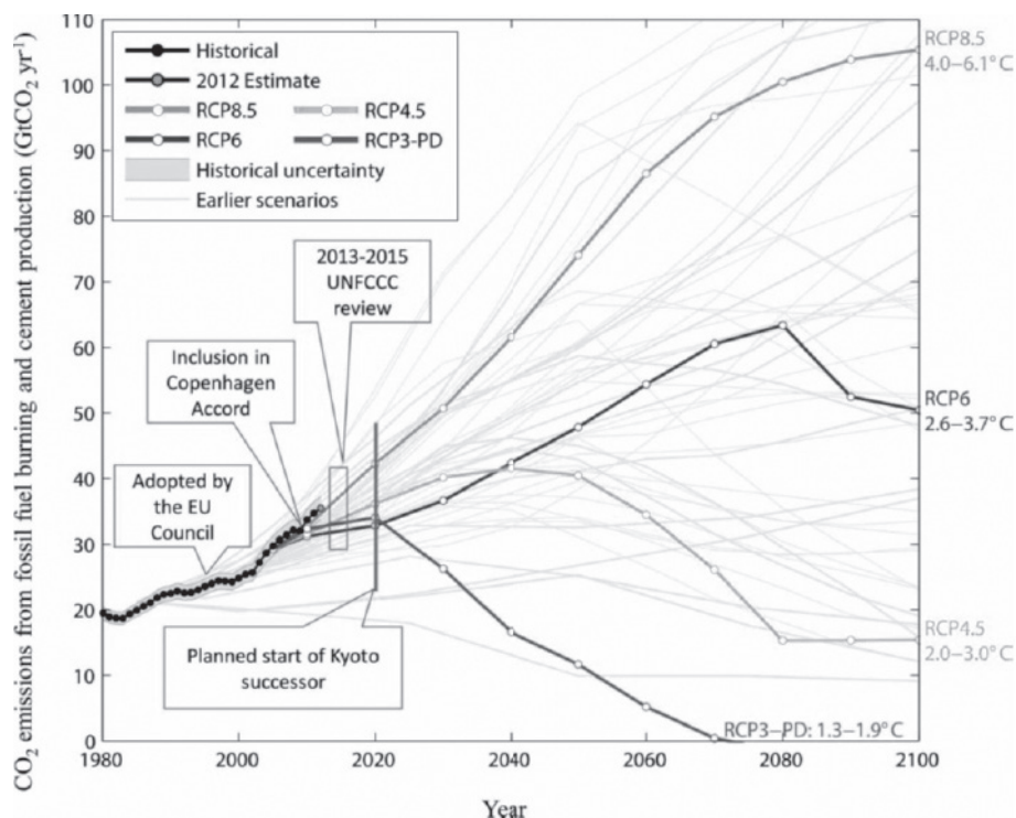
Σχήμα 3: Απεικονίζονται οι καμπύλες των σεναρίων (RCPs) βάσει της εξέλιξης των συνολικών ετήσιων εκπομπών CO 2 -κάθετος άξονας- από το 1980 έως το 2100. Με τις μαύρες κουκίδες απεικονίζεται η εξέλιξη των σημερινών εκπομπών μέχρι την εκτίμηση του 2012 (κόκκινη τελεία), δείχνοντας ότι βαδίζουμε στο χειρότερο δυνατό σενάριο - RCP8,5 -. Στο τέλος κάθε καμπύλης σεναρίου αναγράφεται το εύρος της αναμενόμενης αύξησης της μέσης θερμοκρασίας το 2100. 21
