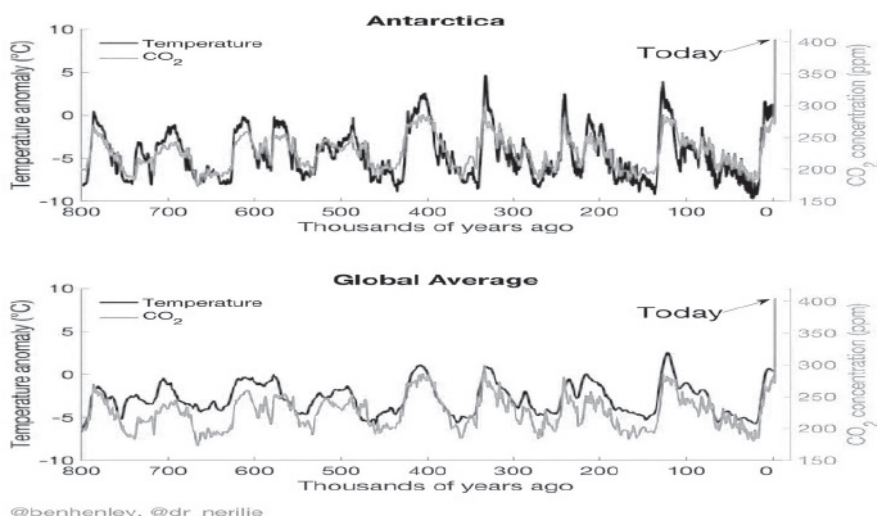
Σχήμα 2: Διακύμανση της μέσης θερμοκρασίας και της μέσης συγκέντρωσης CO 2 στην ατμόσφαιρα τα τελευταία 800.000 χρόνια. Πηγή: Ben Henley & Nerilie Abram. 13
