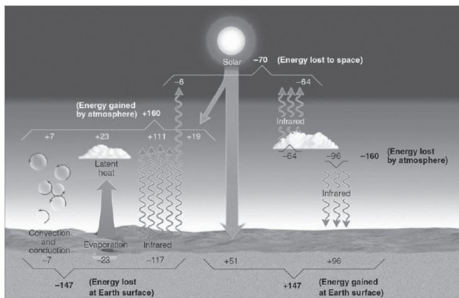
Εικόνα 1. Το ενεργειακό ισοζύγιο του συστήματος Γη-ατμόσφαιρα. Πηγή: Ahrens et al 2016. 9
