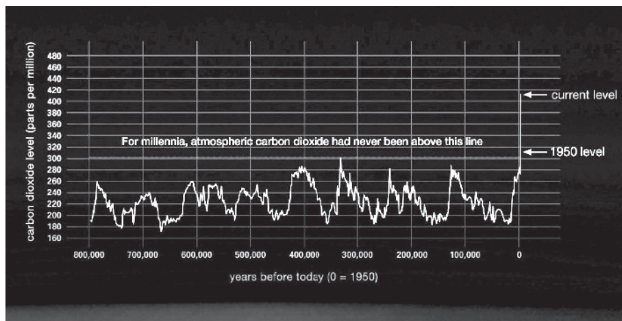
Σχήμα 1: Συγκέντρωση \text{CO}_2 στην ατμόσφαιρα σε ppm τα τελευταία 800.000 έτη. Πηγή NASA. 10
